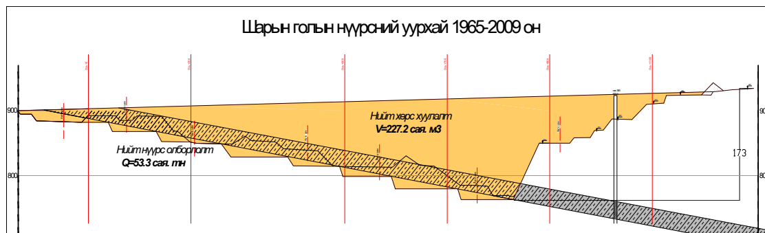
Зураг 3 Одоогийн олборлолт явуулж буй уурхайн хөрс хуулалтын зураг
